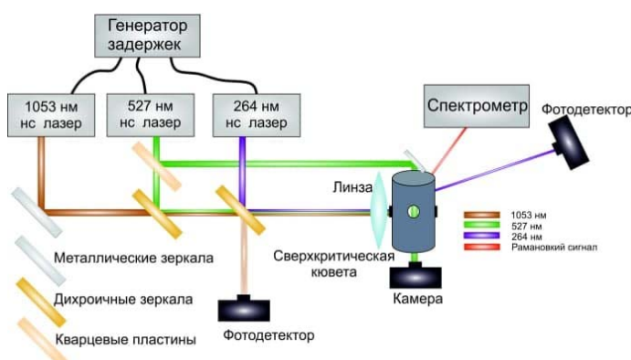
Рис. 1. Система для время-разрешенной диагностики экстремального состояния вещества в сверхкритическом диоксиде углерода
