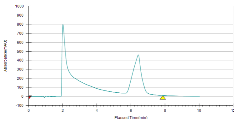
Рис. 1. Хроматограмма разделения салметерола ксинафоата. Условия: ПФ \text{CO}_2/\text{MeOH} 70 : 30, препаративная колонка Chiralpak IG, давление 120 бар, скорость потока 160 г/мин, объем вводимой пробы 2 мл
