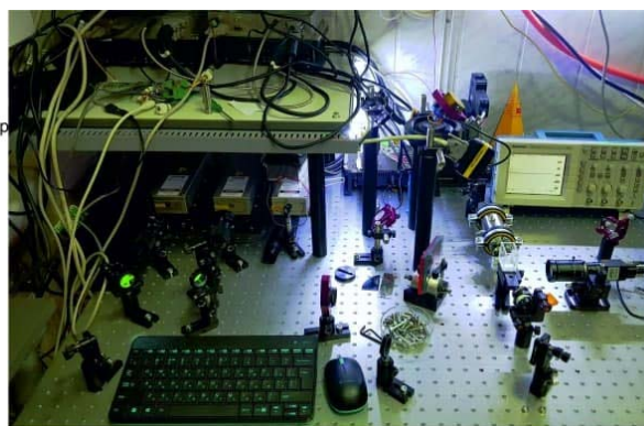
Рис. 1. Система для время-разрешенной диагностики экстремального состояния вещества в сверхкритическом диоксиде углерода
