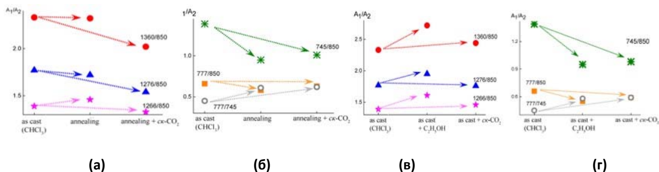
Рис. 1. Изменения относительных интенсивностей полос поглощения функциональных групп ПЭИ в зависимости от способа обработки пленок: а, б – отжиг, отжиг+ск-СО 2 ; в, г – обработка в этаноле и ск-СО 2 .
